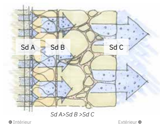
Perméance croissante de l'intérieur vers l'extérieur
