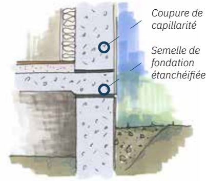
COUPE VERTICALE D'UNE PAROI ÉTANCHE AU NIVEAU DU PLANCHER BAS
