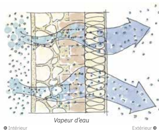
Principe hygrothermique d'une paroi perspirante
