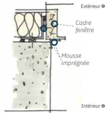
Nouvelle fenêtre posée en prolongement de l'ITE en précadre
