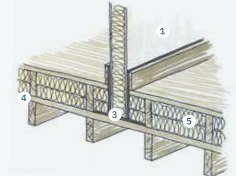
Isoler au dessus des solives
