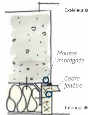
Dépose totale, fenêtre située en tableau sans ébrasement ni feuillure dans le mur
