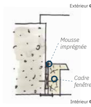
Dépose totale, fenêtre avec feuillure dans le mur
